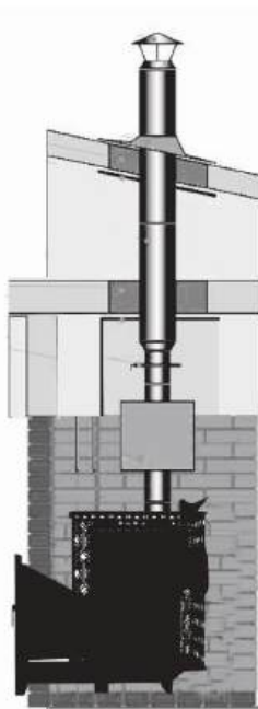
2 вариант установки
