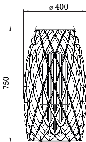
Рисунок 1. Габаритные размеры электрокаменки
