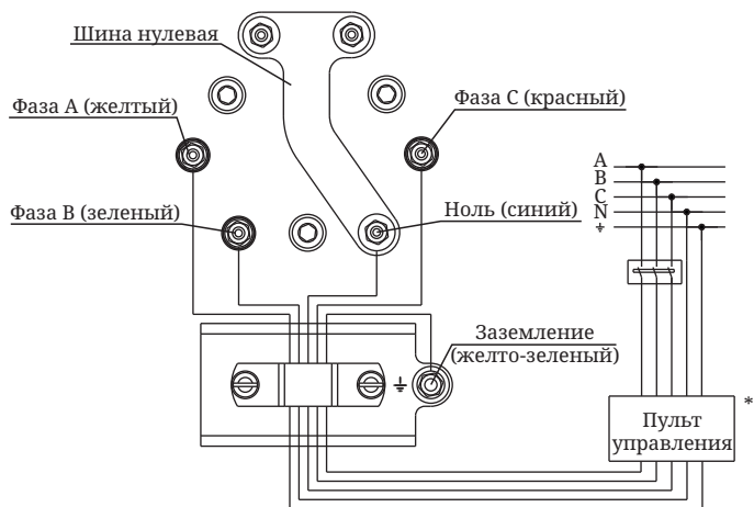
Рисунок 4. Монтажная схема подключения электрокаменки к трехфазной сети.
