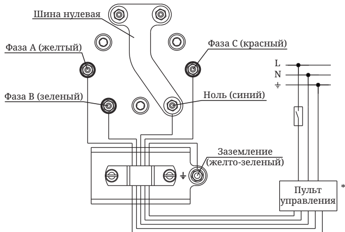
Рисунок 5. Монтажная схема подключения электрокаменки к однофазной сети.
