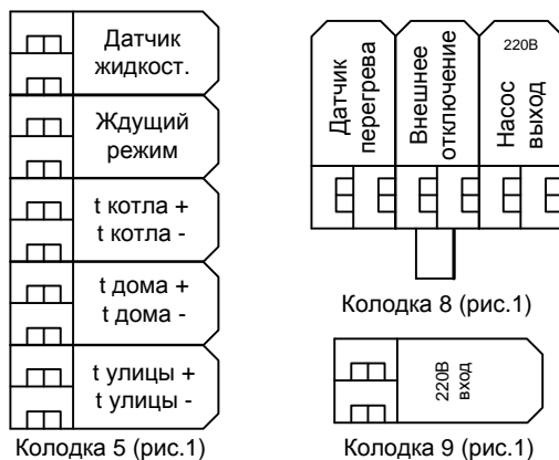
Рисунок б. Колодки подключения внешнего оборудования
