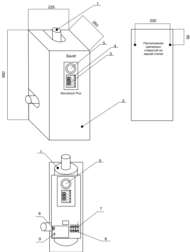
Рис.1 Общий вид изделия типа «Monoblock Plus».
