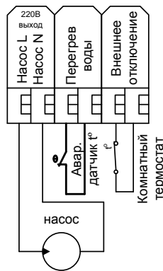
Рисунок 5. Колодка подключения внешнего оборудования
