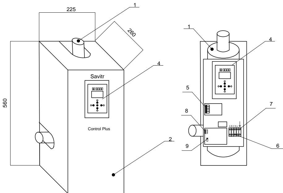
Рис.2 Общий вид изделия модели «Control Plus».
