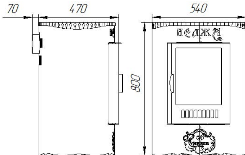
Рисунок 2. Общий вид печи, с нанесенными основными размерами .
